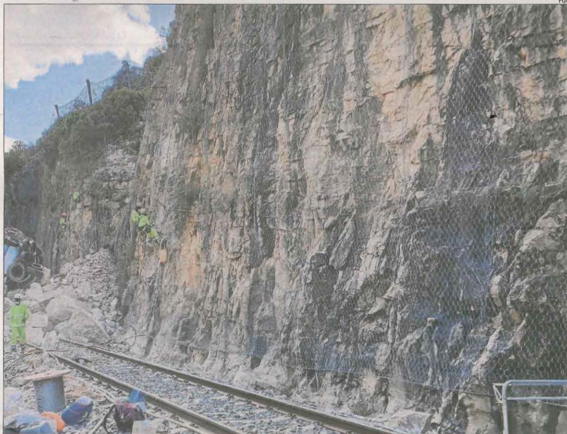
Els operaris treballen directament sobre el talús per estabilitzar les roques.
